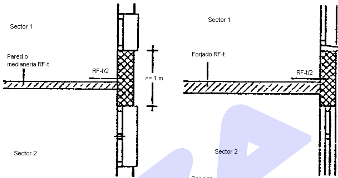
Planta Encuentro de una pared o medianería con la fachada
